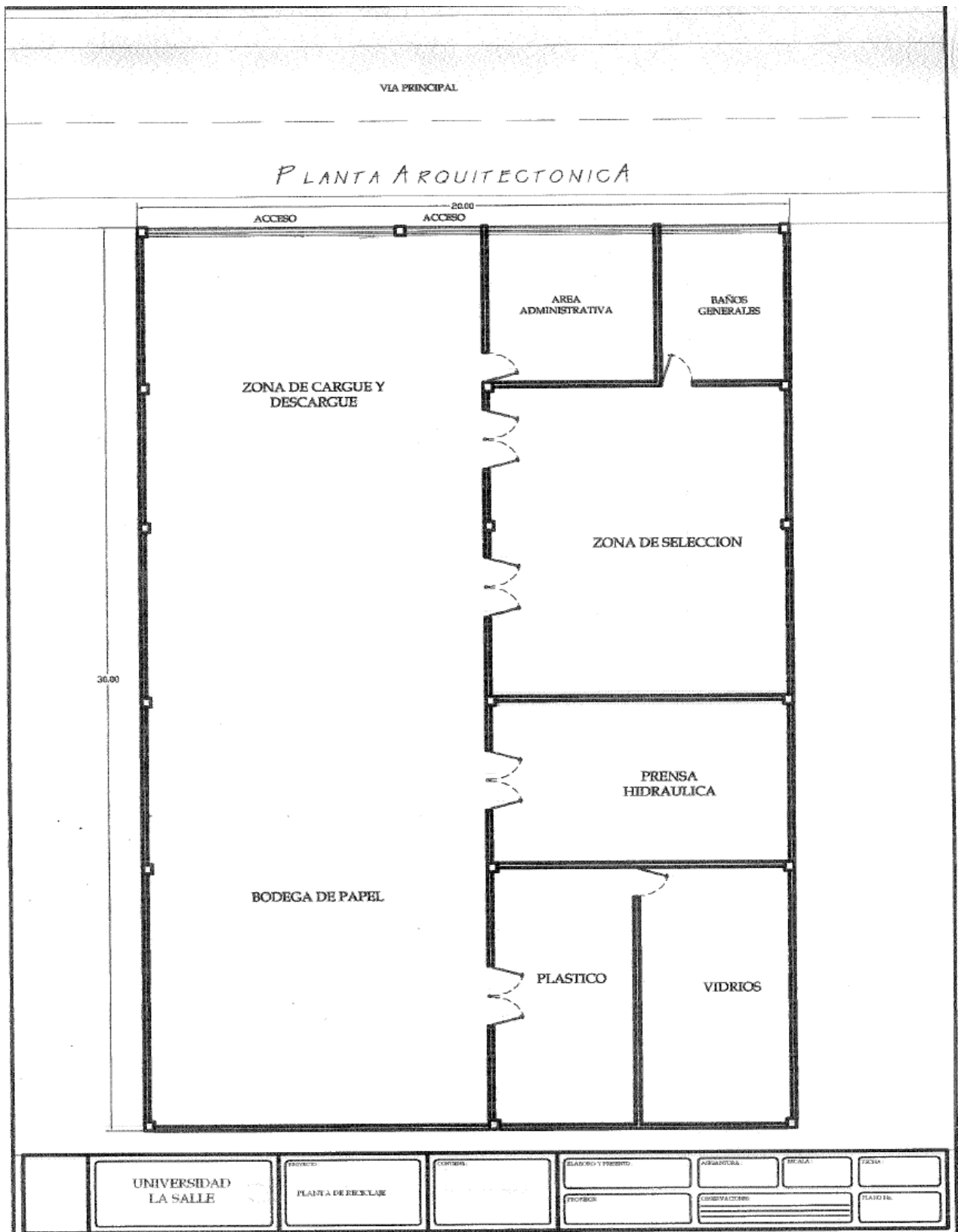
Figura 3. Diseño de la planta de reciclaje
